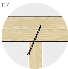
Verbindung Stiel-Randbalken mit einem geneigten Verbinder
