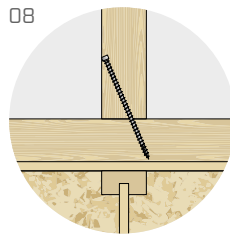
Verbindung Stiel-Randbalken mit einem geneigten Verbinder
