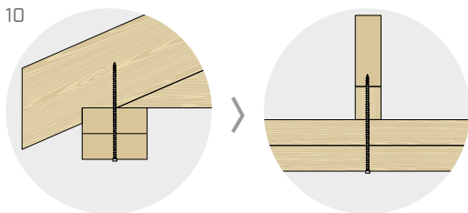
Verbindung Obergurt-Sparren-Randbalken mit einem geneigten Verbinder
