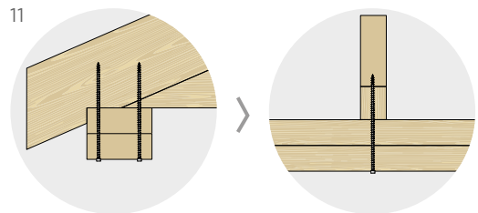
Verbindung Obergurt-Sparren mit zwei vertikalen Verbindern
