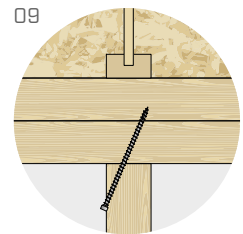
Verbindung Stiel-Randbalken mit einem geneigten Verbinder
